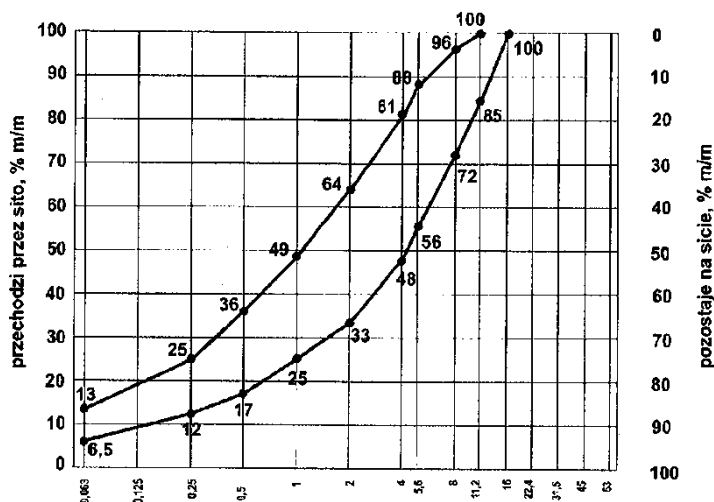
Rys. 4. Krzywe graniczne uziarnienia mieszanki mineralnej 0/11,2 mm
