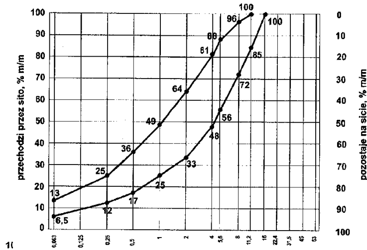
Rys. 3. Krzywe graniczne uziarnienia mieszanki mineralnej 0/16 mm
