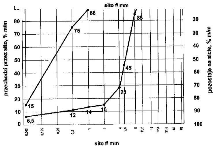
Rys. 4. Krzywe uziarnienia mineralnej 0/11,2
