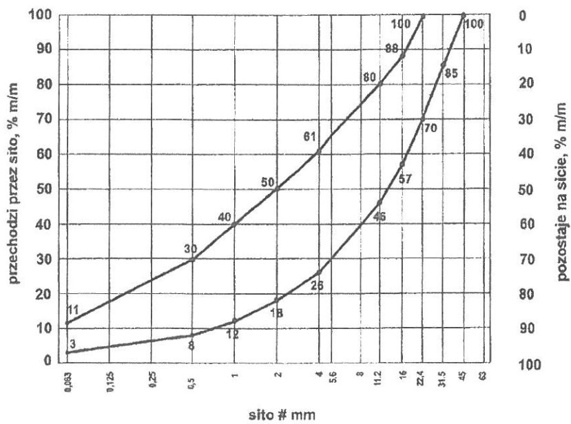
Rys. 1. Krzywe graniczne uziarnienia mieszanek mineralnej 0/31,5 mm
