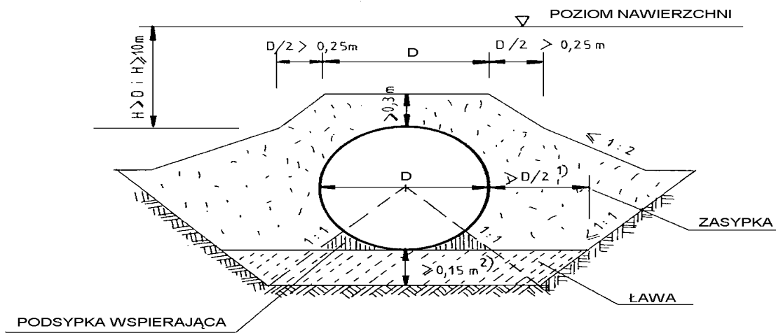
Rys. 8. Zasyпка nad przepustem jednorurowym
