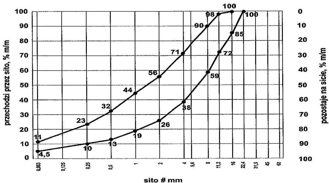
Rys. 3. Krzywe graniczne uziarnienia mieszanki mineralnej 0/16 mm
