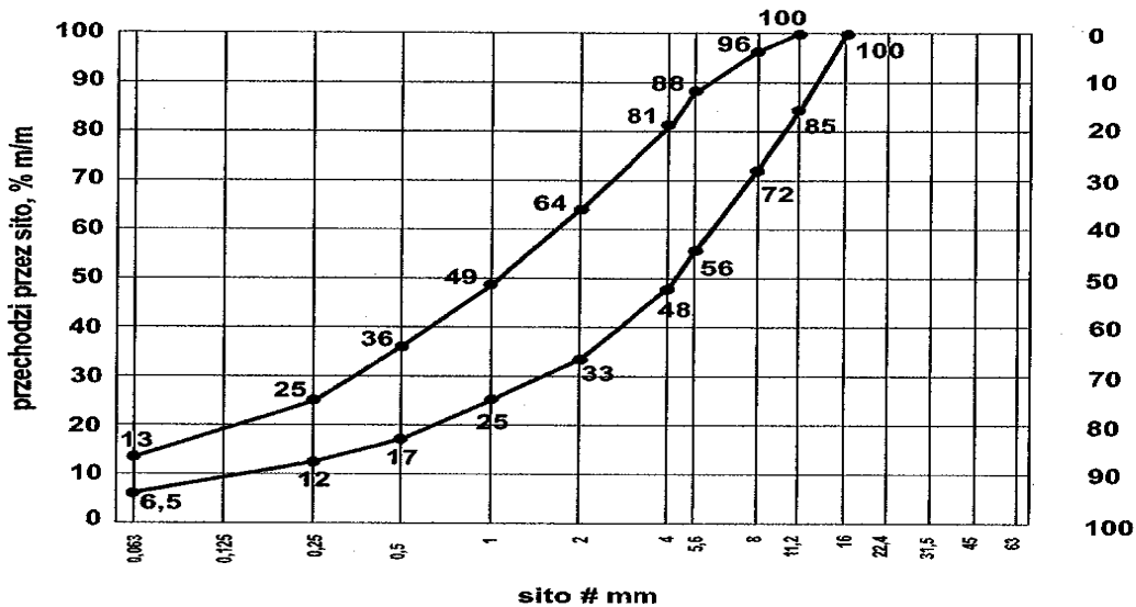
Rys. 4. Krzywe graniczne uziarnienia mieszanki mineralnej 0/11,2 mm
