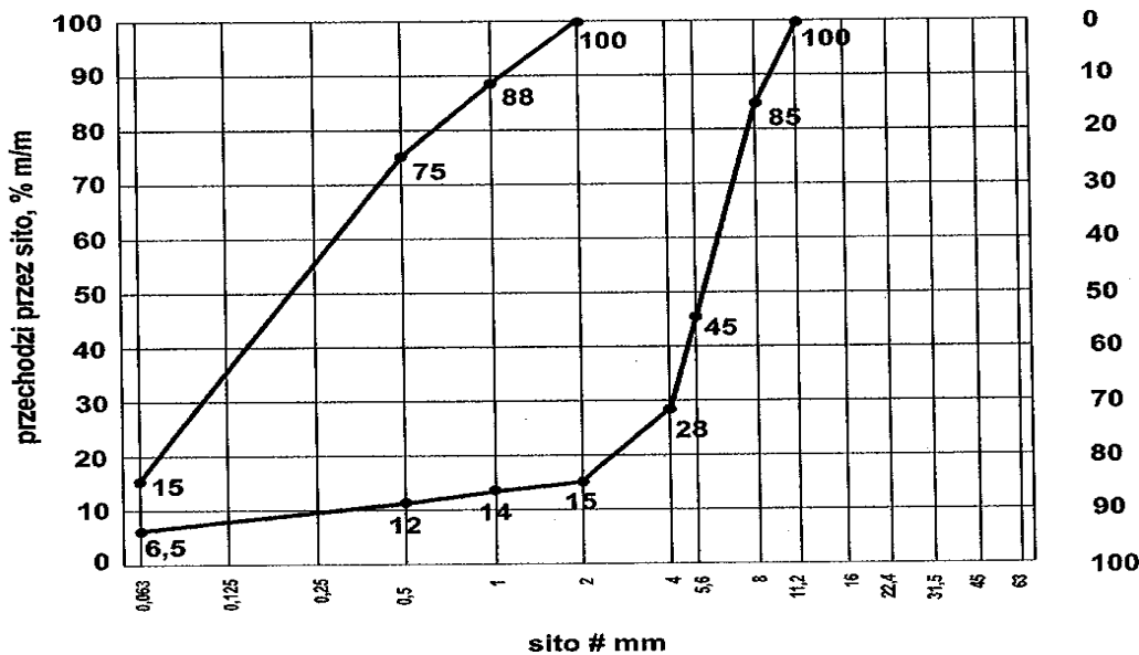
Rys.5. Krzywe graniczne uziarnienia mieszanki mineralnej 0/8 mm
