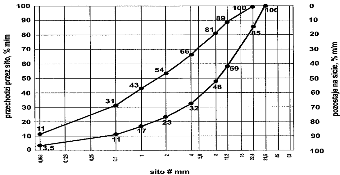
Rys. 2. Krzywe graniczne uziarnienia mieszanki mineralnej 0/22,4 mm
