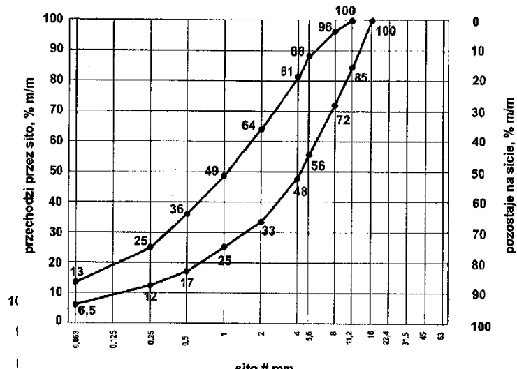
Rys. 3. Krzywe graniczne uziarnienia mieszanki mineralnej 0/16 mm
