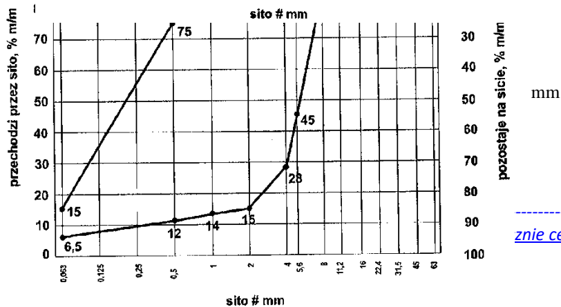
Rys. 4. Krzywe uziarnienia mineralnej 0/11,2
